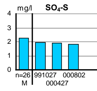
Figur 6. Depositions- och markvattendata från Mellan Hurr, S 16.
