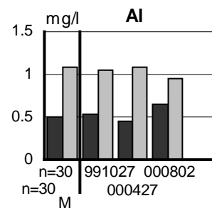
Figur 4. Depositions- och markvattendata från Södra Averstad, S 05.
