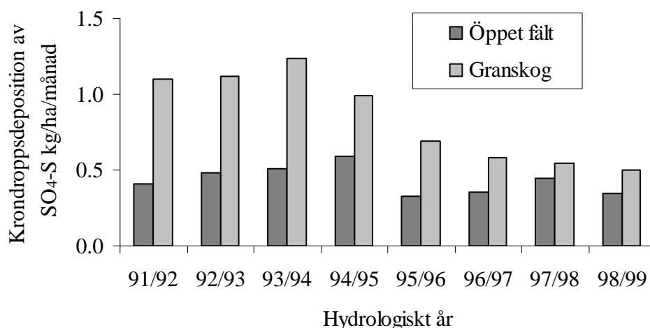
Figur 14. Deposition av sulfatsvavel i granskog (kronddropp) och på öppet fält i en provyta med medelålders gran i Asa försökspark.
