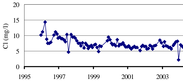
Figur 18. Kloridkoncentration i huvudfåran, bäck LIV3. Kloridkoncentrationen minskade signifikant från december 1995 till april 2004.
