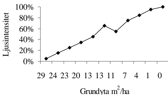
Figur 11. Ljusintensitet som funktion av grundyta. Notera att det finns två klasser med grundytan 13 m 2 per hektar.
