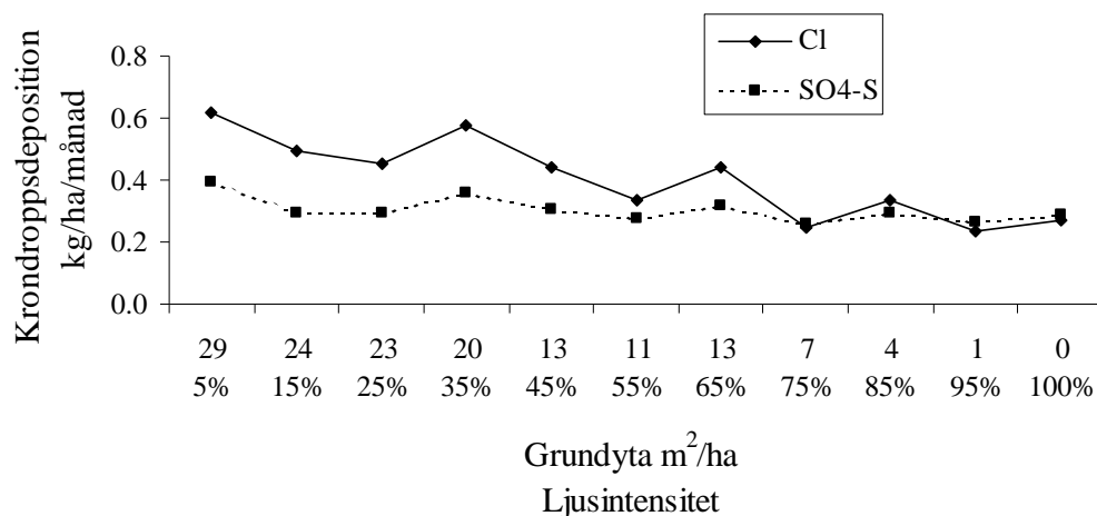
Figur 13. Klorid och sulfatsvavel i kronddropp som funktion av skärmtätheten. Notera att det finns två klasser med grundytan 13 m 2 per hektar.
