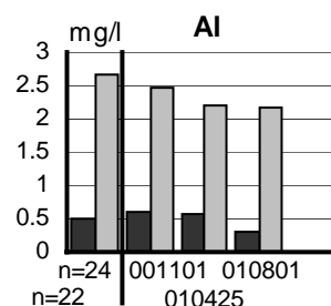
Figur 7. Deposition och markvattendata från Kvisterhult, U 04.
