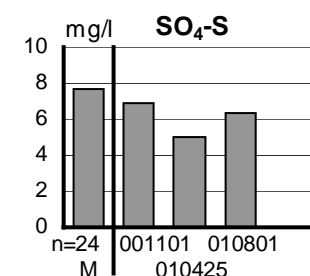
Figur 7. Deposition och markvattendata från Kvisterhult, U 04.
