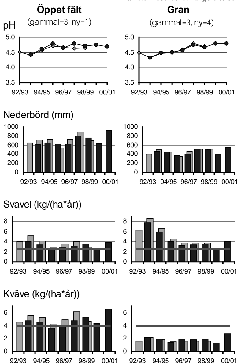
Figur 10. Årsmedelvärden för valda parametrar i två miljöer i Västmanland; öppet fält och granskog, uppdelat på två delvis överlappande tidsserier. Figuren visar tidsutvecklingen trots övergång från "gammal" serie (från 1992/93) till "ny" serie (från 1993/94) Streckad linje anger genomsnittlig förväntad nivå år 2010 i Svealand om beslutade åtgärder genomförs (se sid. 3).
