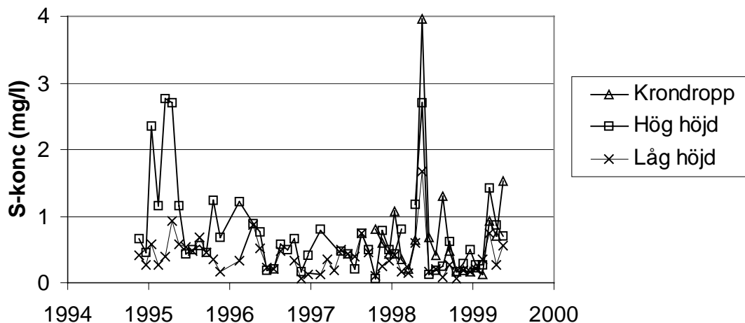
Figur 1. Uppmätt svavelhalt på Sånfjället (Z910), månadsvärden.
