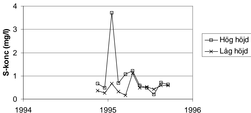
Figur 2. Uppmätt svavelhalt i nederbörd på Skorvfjället (Z920).
