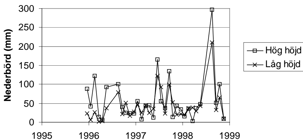
Figur 10. Uppmätt nederbördsmängd på Härjångstöten (Z940), månadsvärden.
