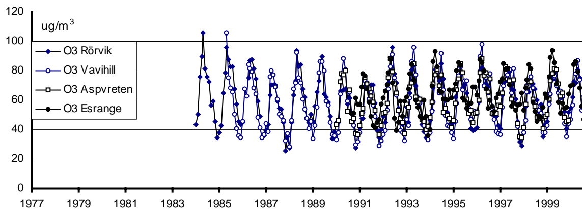
Figur 15. Månadsmedelvärden av svaveldioxid, (SO 2 ) kvävedioxid (NO 2 ) och ozon (O 3 ) på fyra EMEP-lokaler i Sverige; Vavihill i centrala Skåne, Rörvik söder om Göteborg, Aspvreten öster om Nyköping samt Esrange öster om Kiruna. Observera att stationernas mätningar startar olika år och att det är annan skala än i figur 14.
