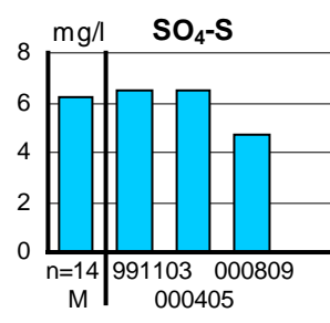
Figur10. Depositions- och markvattendata från Angelstad, G 23.
