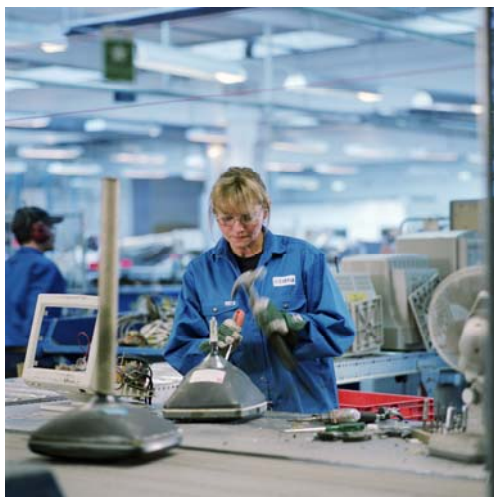
Figur 4.2 Demontering av CRT.
