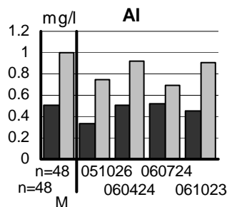
Figur 3. Depositions- och markvattendata från Södra Averstad, S 05.
