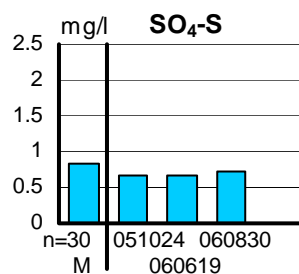
Figur 5. Depositions- och markvattensdata från Transtrandsberget, S 23.
