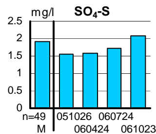
Figur 3. Depositions- och markvattendata från Södra Averstad, S 05.
